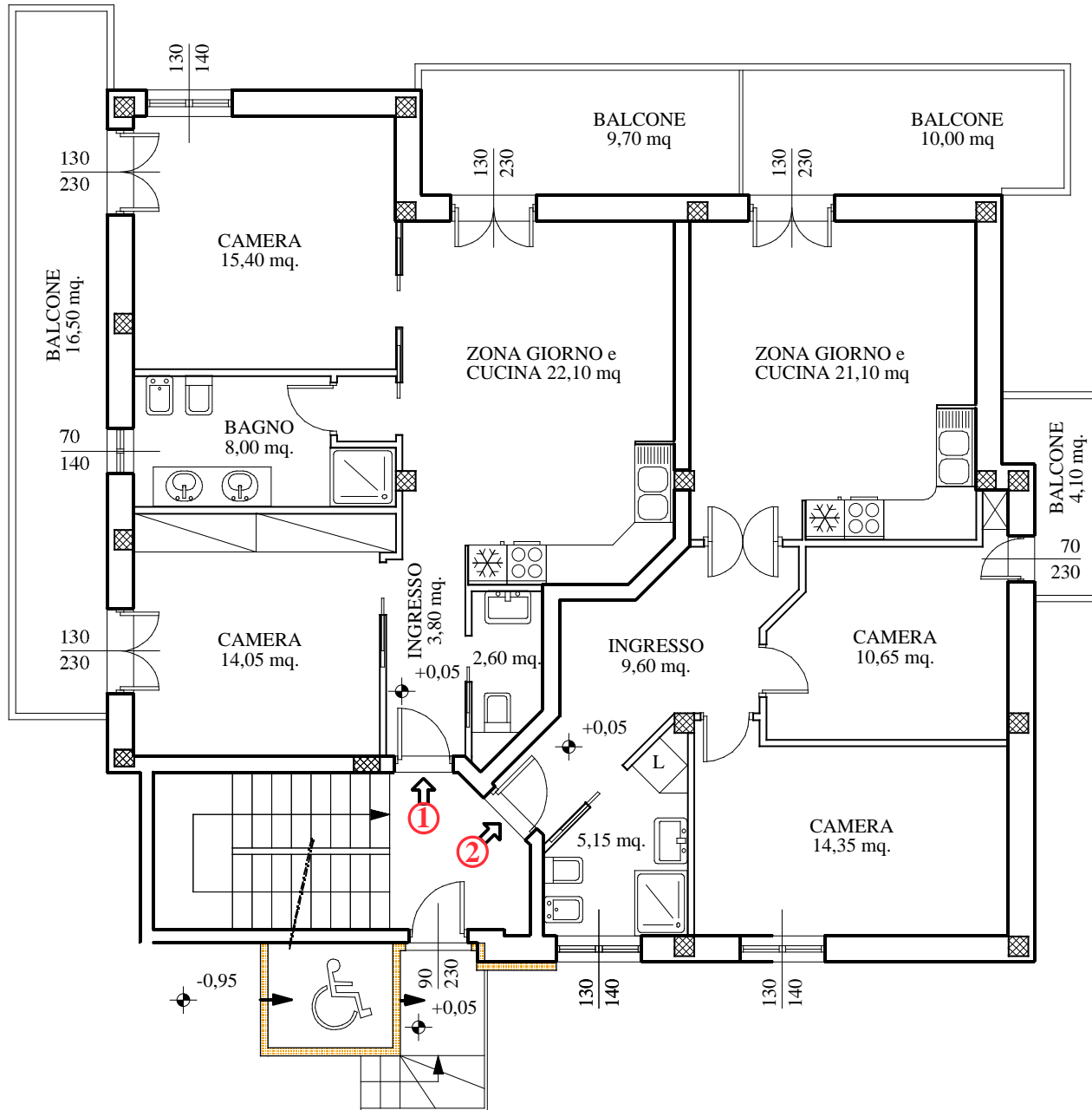
Pianta Piano Terreno - Progetto -
