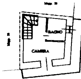
PIANO SECONDO H = 2.40
