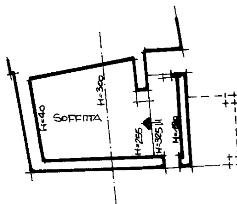
PIANO SOTTOTETTO (SECONDO)
